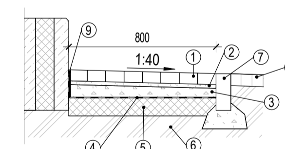
LÕIGE 1-1 (1 : 20)
