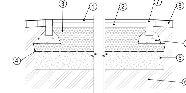
LÕIGE 2-2 (1 : 20)
