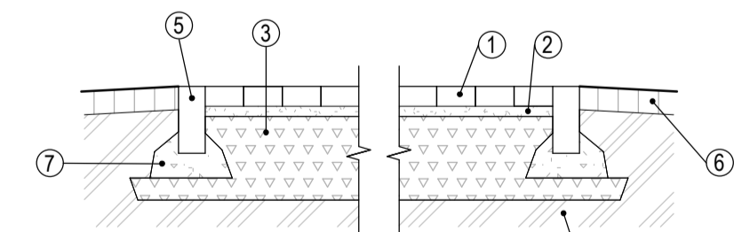
LÕIGE 3-3 (1 : 20)
